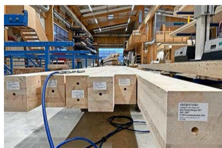
Die Elemente der Holzkonstruktion wurden passgenau vorproduziert. BILD GF
