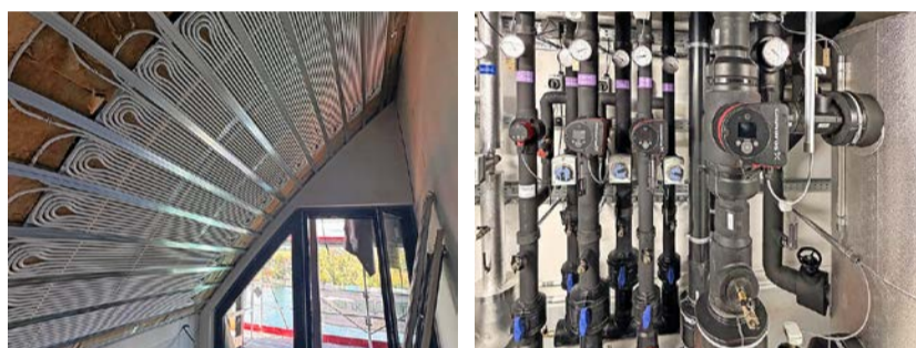
Die Kühlung ist unter einer Gipslochdecke verborgen (l.). Im Keller wird warmes und kaltes Wasser in Tanks gespeichert, die jeder 2000 Liter fassen (r.).
